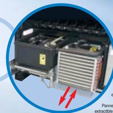
Portillon produit mono-bloc facilement extractible pour l'accès au groupe froid.
