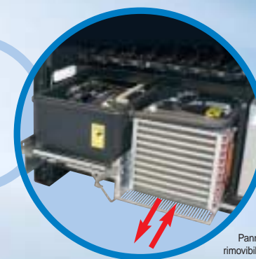
Parte interna della tasca prelievo mono-blocco, facilità di rimozione per raggiungere il gruppo frigo.
